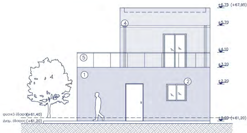
ΒΟΡΕΙΑ ΟΨΗ
