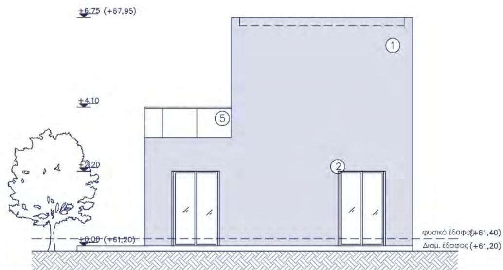
ΒΟΡΕΙΑ ΟΨΗ
