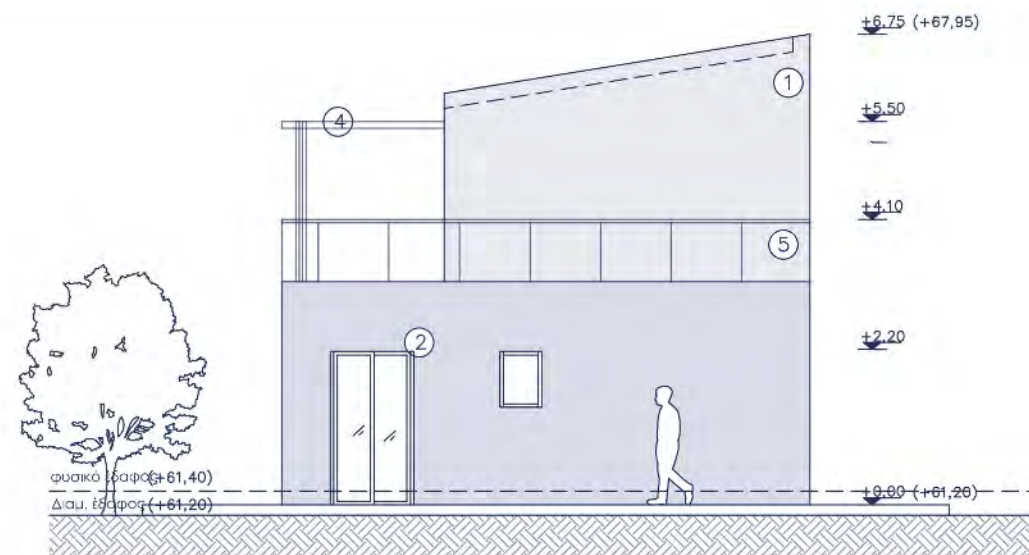
ΑΝΑΤΟΛΙΚΗ ΟΨΗ
