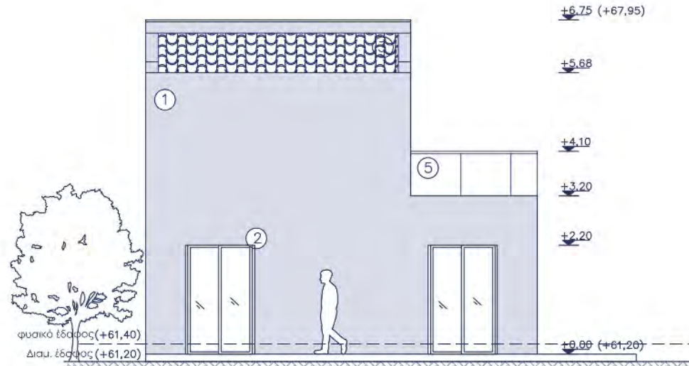
ΝΟΤΙΑ ΟΨΗ
