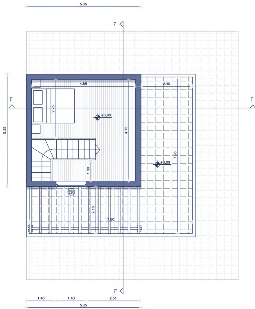
ΚΑΤΟΨΗ ΣΟΦΙΤΑΣ 28 τ.μ.
