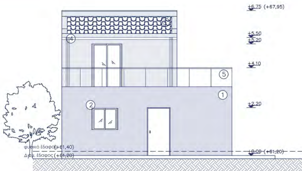
ΝΟΤΙΑ ΟΨΗ
