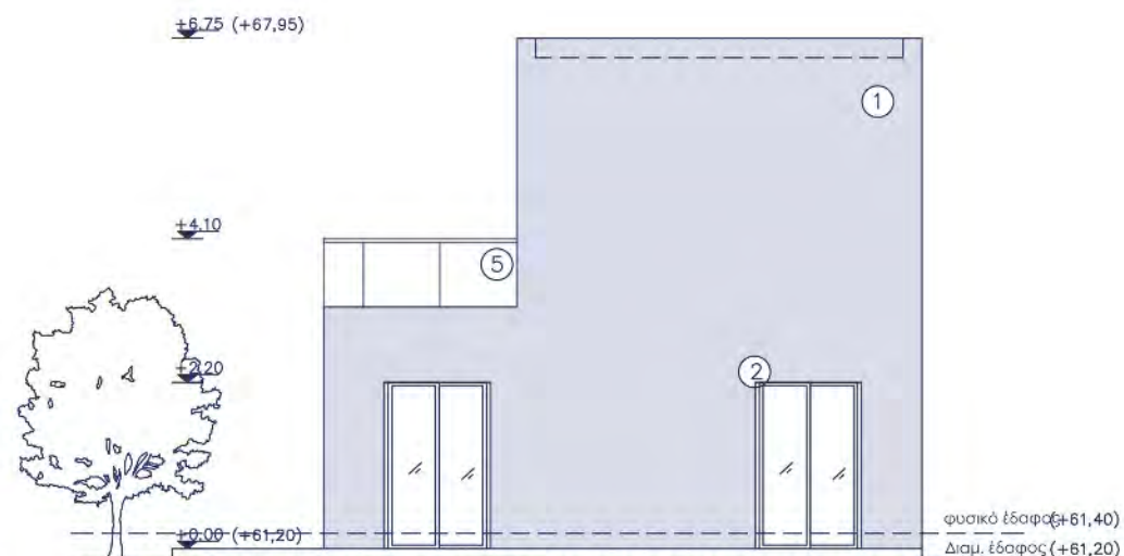
ΒΟΡΕΙΑ ΟΨΗ
