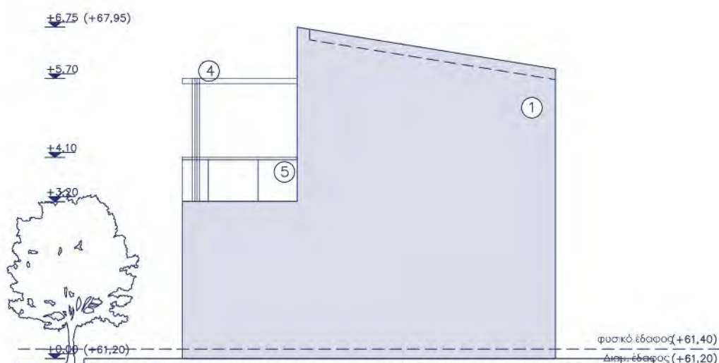
ΔΥΤΙΚΗ ΟΨΗ
